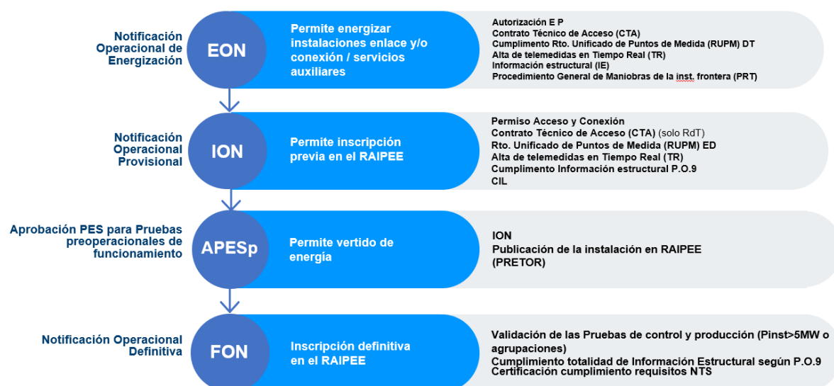
Figura 4. Notificaciones operacionales aplicables a instalaciones de enlace y conexión, y MGE conectados a RdT
