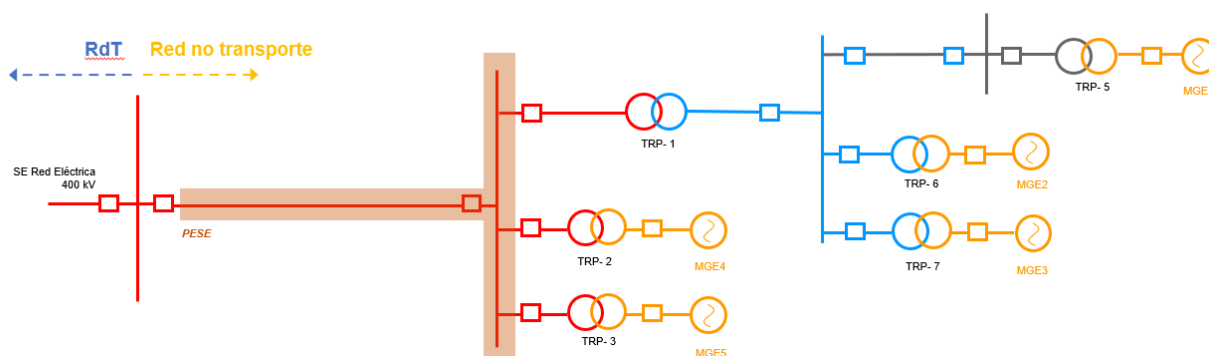
Figura 5. Ejemplo de instalación de enlace y solicitud PESE
