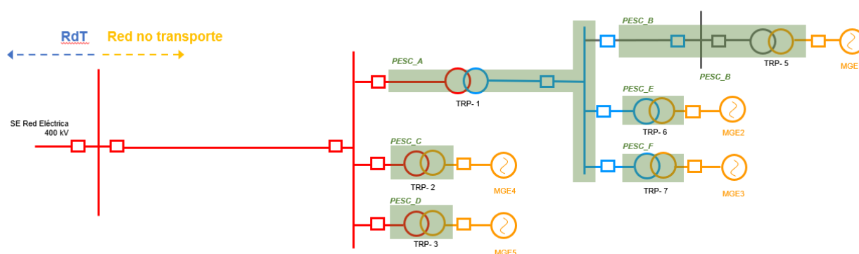
Figura 6. Ejemplo de instalaciones de conexión y solicitudes PESC
