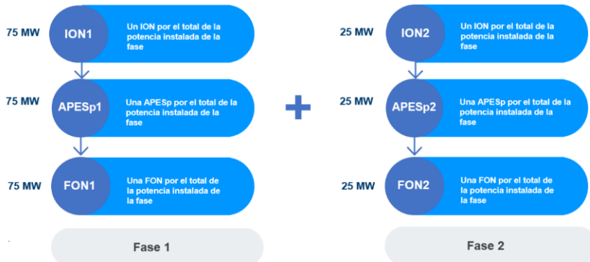
Figura 10. PES en dos fases (75MW y 25 MW) con APESp total en ambos casos.
