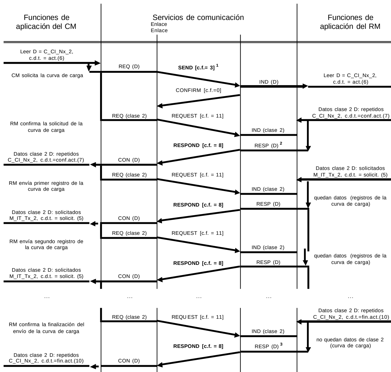
Figura 5-1: Transmisión de totales integrados (curva de carga)
