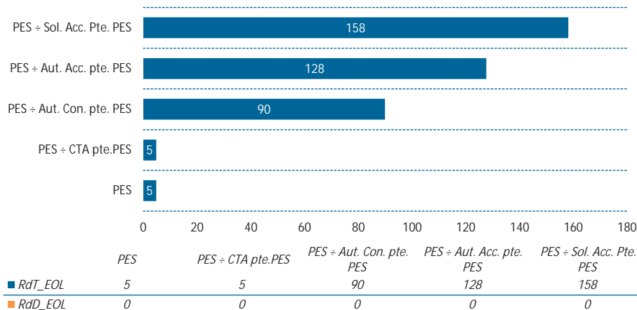
Generación Eólica (MW)
